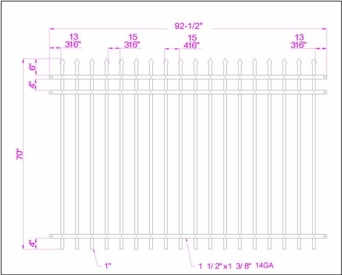
6'H X 8'L LARAMIE PRESSED POINT PICKET
