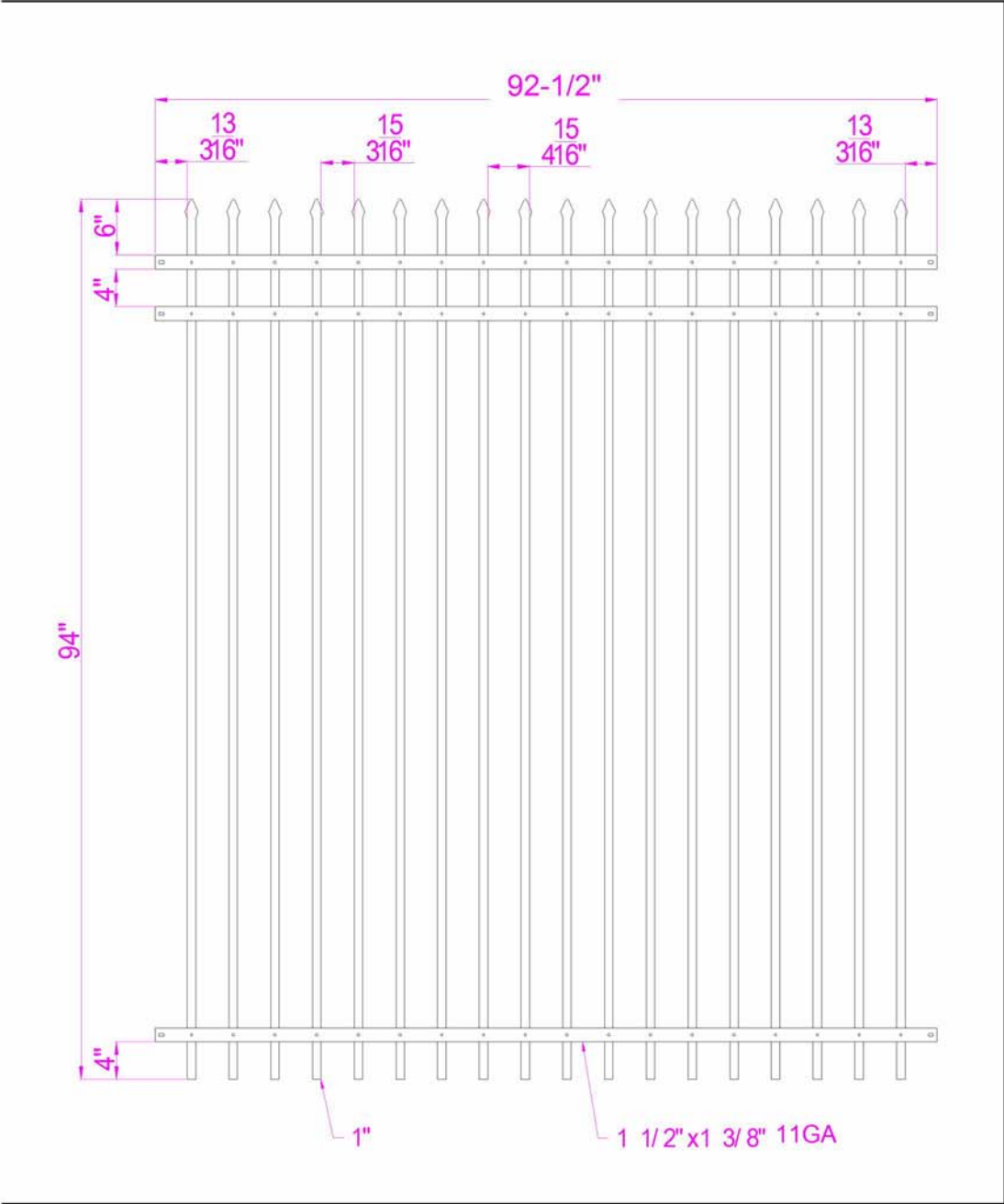
8'H X 8'L LARAMIE PRESSED POINT PICKET
